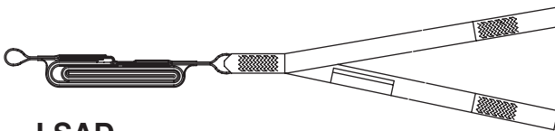
LSAD
